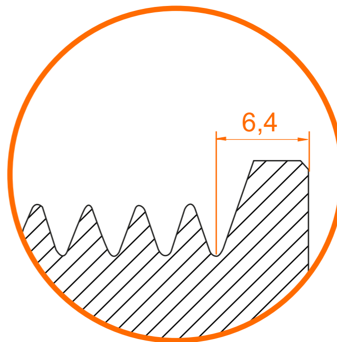
DETALHE DA DISTÂNCIA DO EIXO
